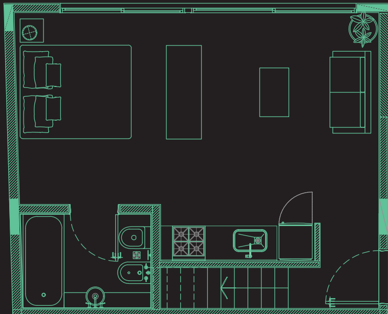
PLANTA BAJA
